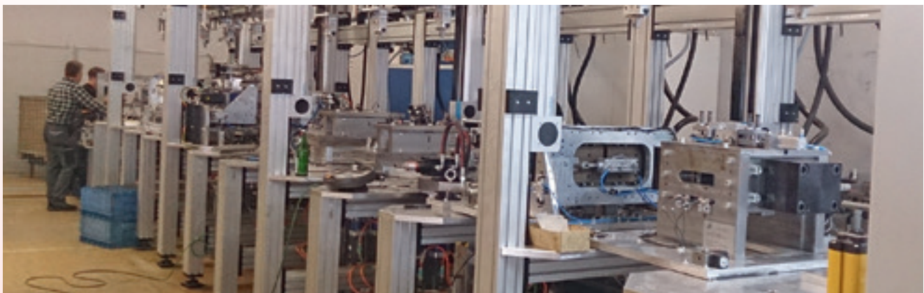
Die in Cobbenrode geplante und gebaute fertige Transferanlage steht bereits bei einem Automotive- Hersteller in Sundern und produziert vollautomatisch 2 Mio. Mercedes- Kopfstützen pro Jahr
